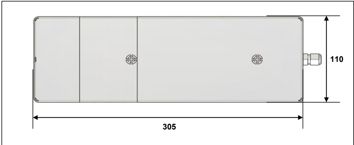
Abbildung 4 Maße des AG300, Draufsicht (Angaben in mm)
